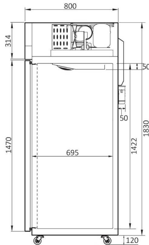
ВИД СБОКУ
